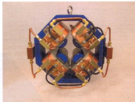
Quadrupole Magnet
